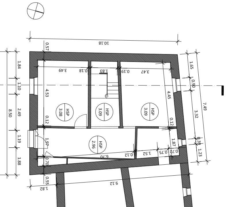
PLAN NIVEAU RDC / 50.22 NGF
