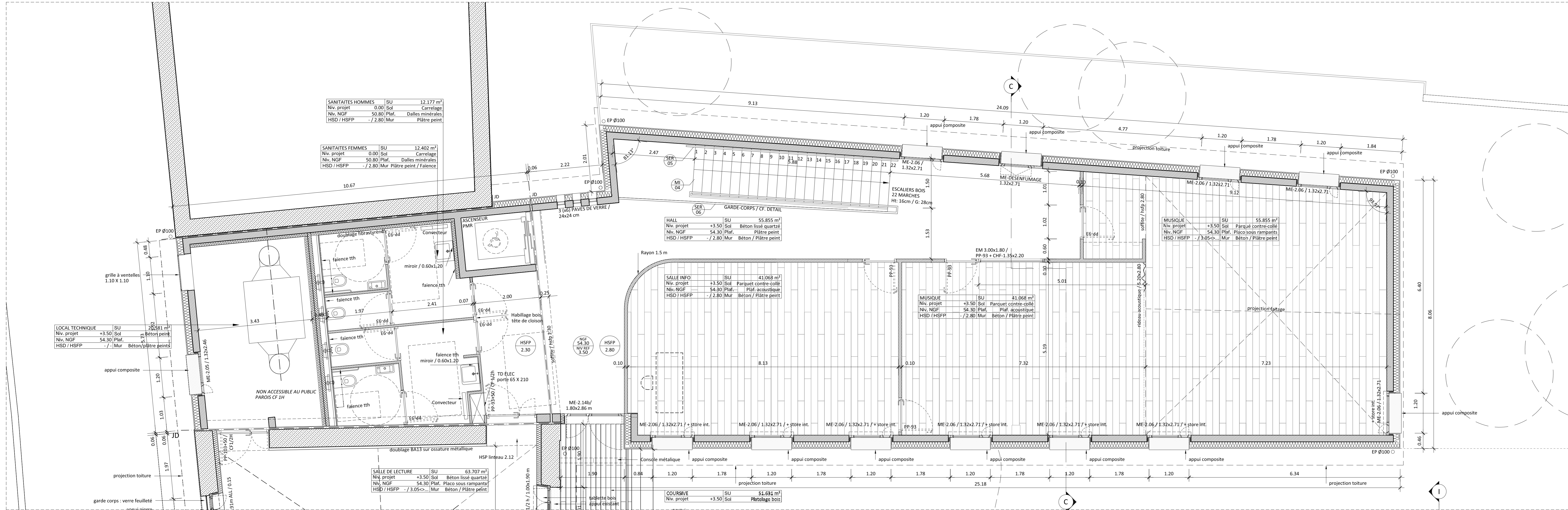
PLAN DU R+1 1/50e
