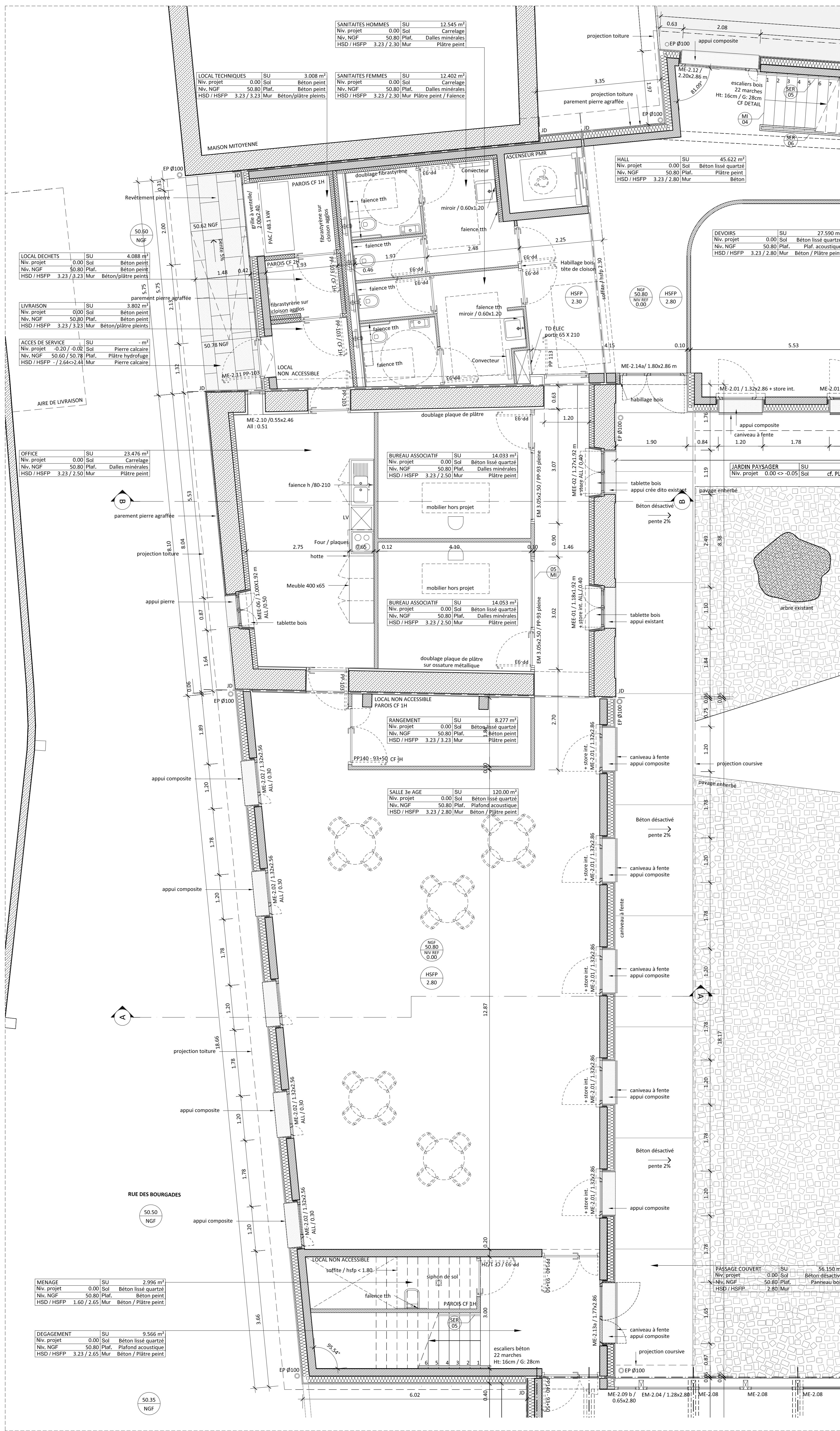
PLAN DU RE-ZE-CHAUSSEE 1/50e
